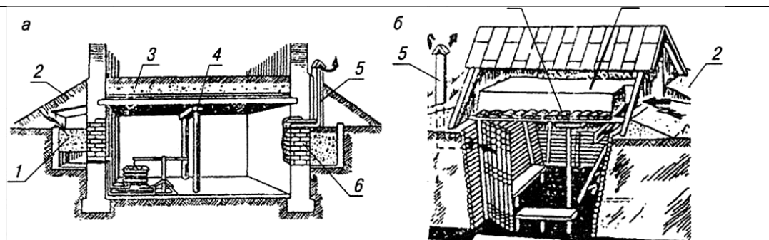
Рис. 2. Оборудование подвального помещения (а) и погреба (б) под противорадиационное укрытие:
