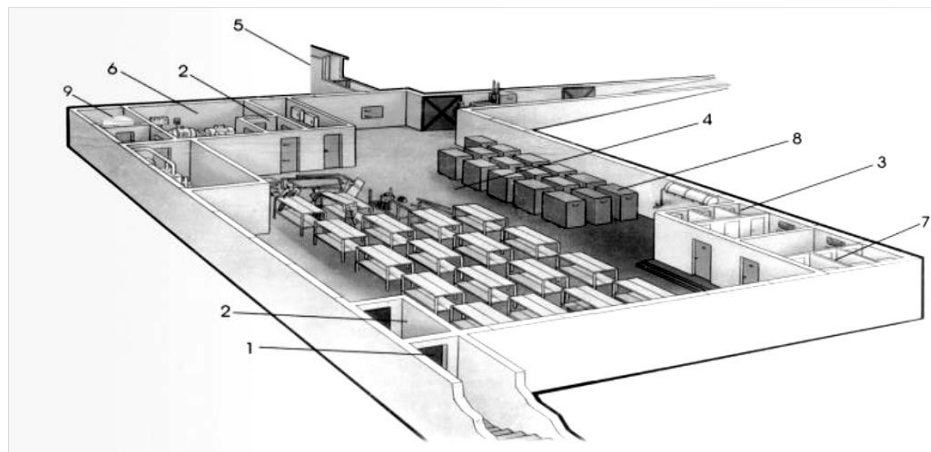
Рис.1 План-схема встроенного убежища
